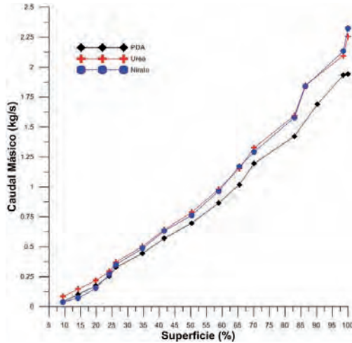
Figura 21. Caudal máximo en función de la superficie de apertura de los tres principales abonos utilizados en el cultivo de cereal: Fosfato diamónico "PDA", Urea y Nitrato amónico "Nitrato"
