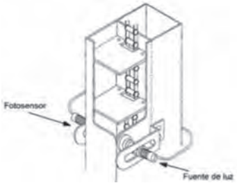
Figura 13. Sistema de medida de rendimiento mediante fotosensores que miden el volumen de grano que pasa instantáneamente.
